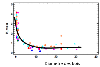
Figure n° 3. Concentration en potassium des bois
