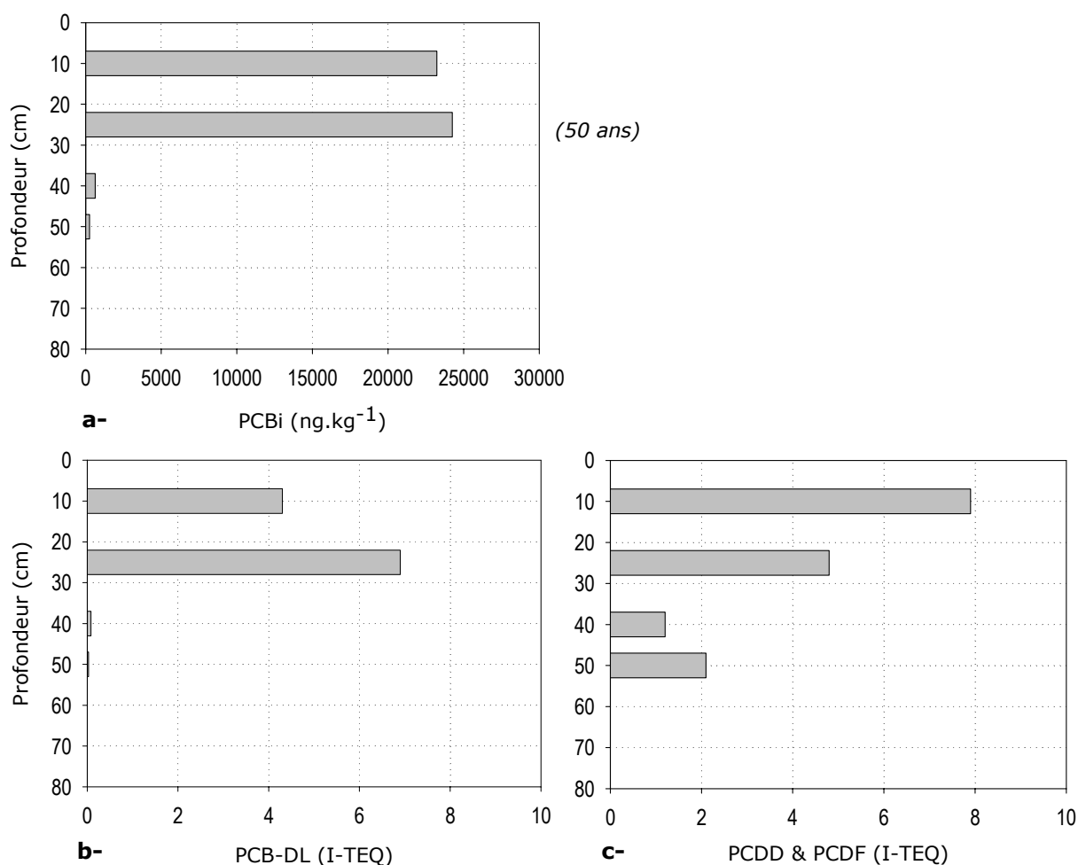
Figure 6 - Profils en profondeur des PCBi, PCB-DL et PCDD et PCDF en GL3
