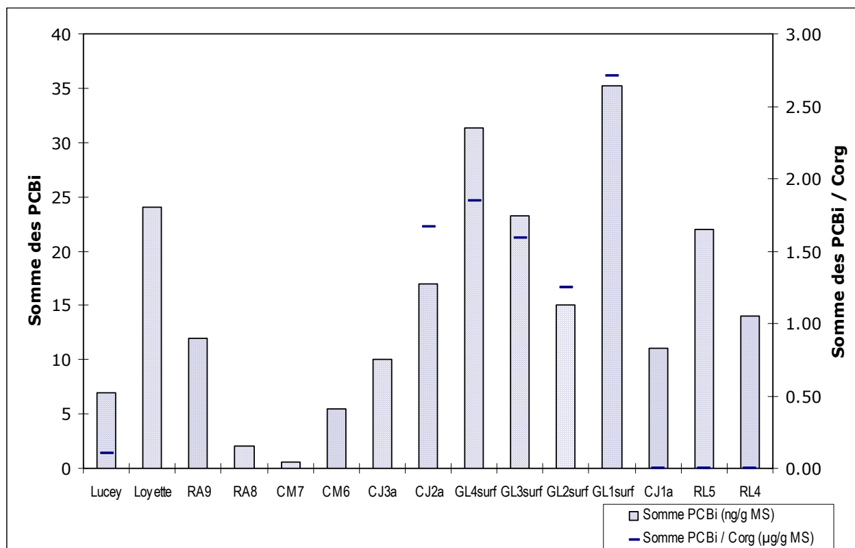
Figure 3 - Analyses de PCBi dans les sédiments superficiels (les concentrations normalisées n'ont été calculées que pour les sites où COT \geq 1%)
